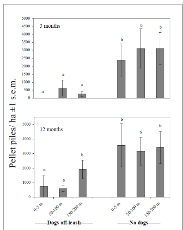
Fig. 2. Densités des crottes de lapins sur 12 mois et 3 mois selon la politique relative aux chiens et la distance par rapport au sentier.
